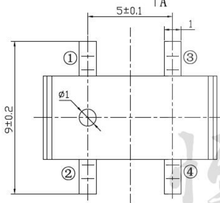
A向
