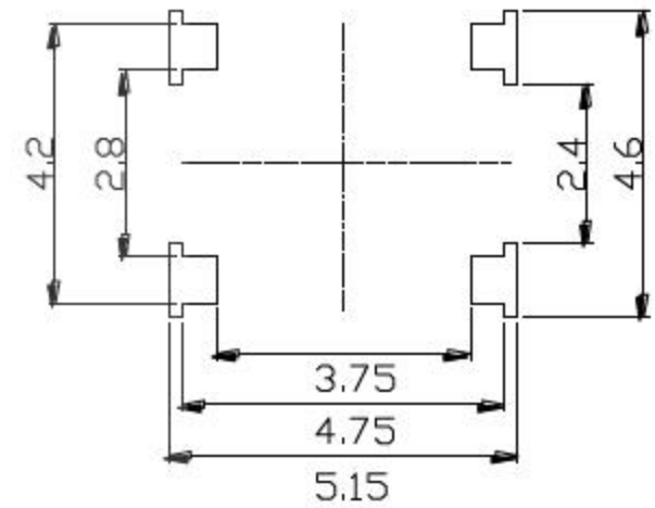
PCB. 焊接图
