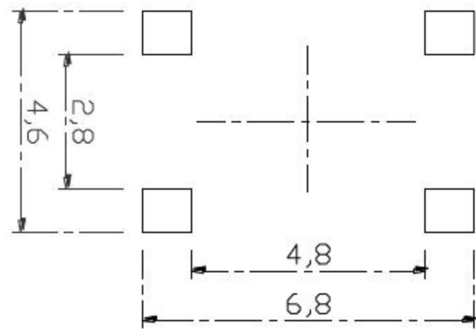
PCB. 焊接图
