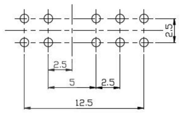
P.C.B LAYOUT
