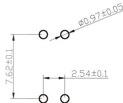
PCB开孔
