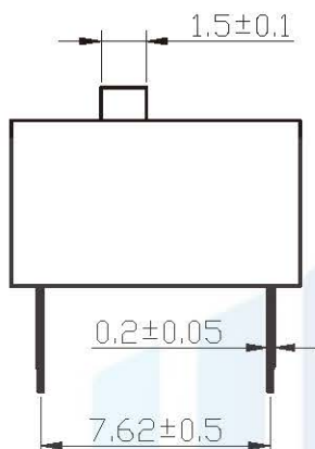
高推钮 (E)
